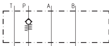
HROP 消耗裝置的壓力夾緊
