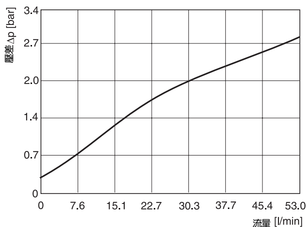
CM2 ( \Delta p/Q -特性曲綫)
