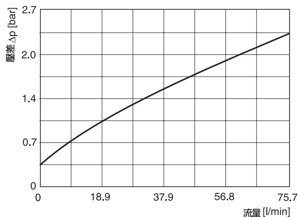
CM3 ( \Delta p/Q -特性曲綫)
